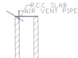
SOAK PIT
