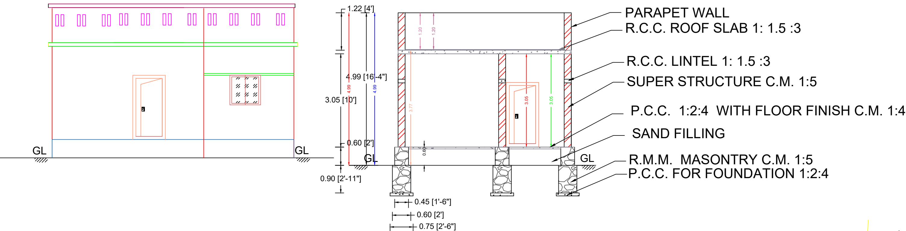
ELEVATION
