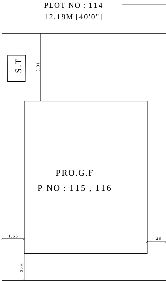
PLOT NO : 117 SITE PLAN SCALE 1:100
