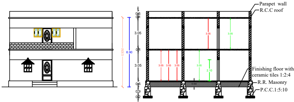
ELEVATION
