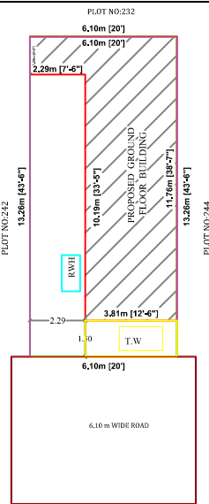
SITE PLAN SCALE 1:100
