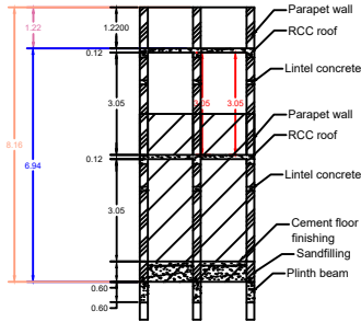
SECTION - AB
