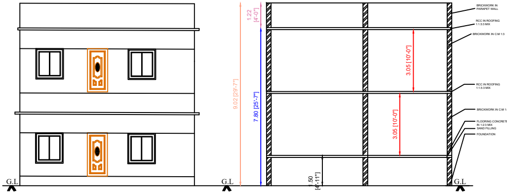
ELEVATION
