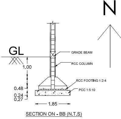
SECTION ON - BB (N.T.S)
