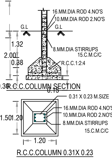
R.C.C COLUMN 0.31X 0.23
