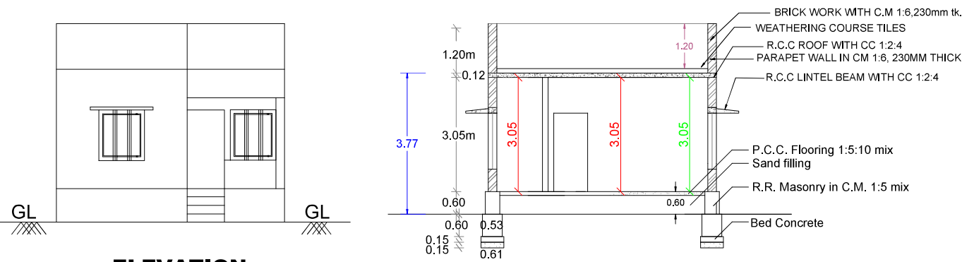
ELEVATION
