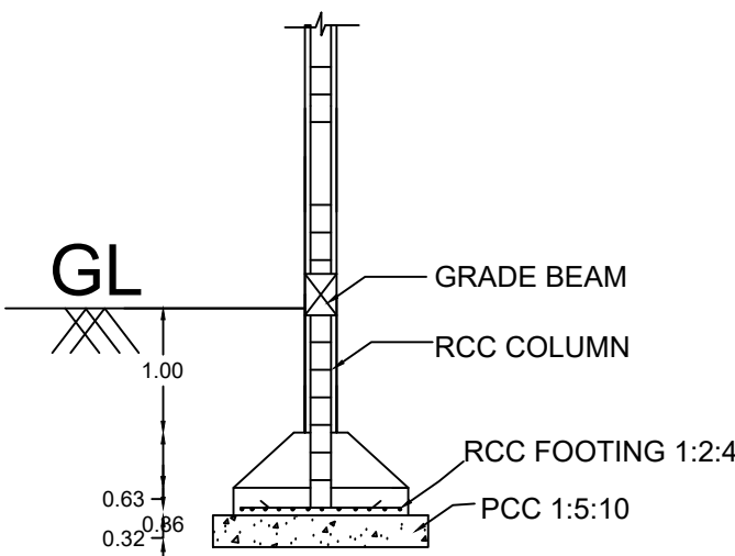
SECTION ON - BB (N.T.S)
