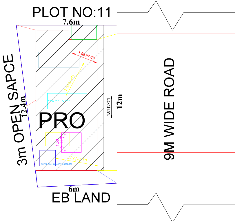
SITE PLAN(SCALE 1:100)
