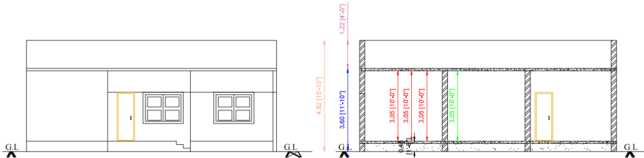
ELEVATION
