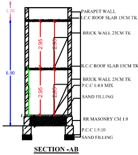
SECTION -AB
