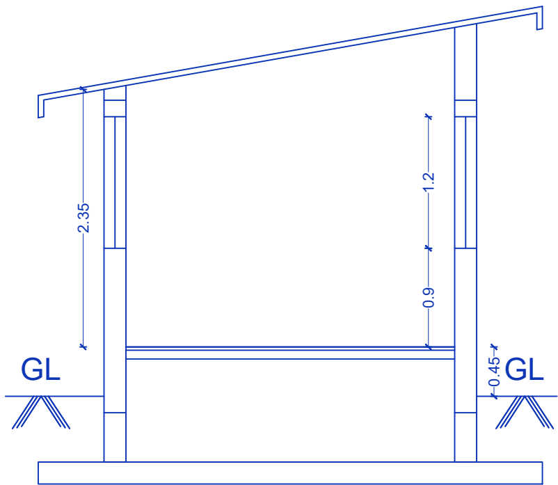
SECTION-A
