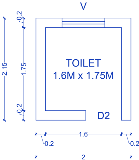
TOILET PLAN
