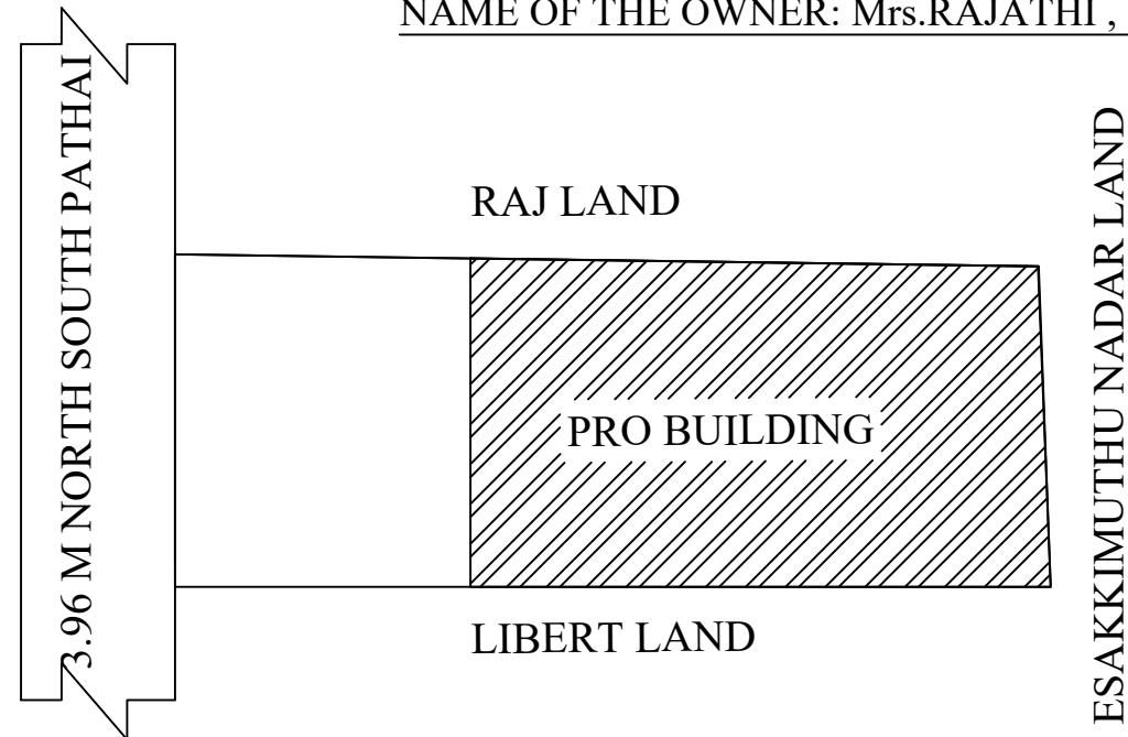
SITE PLAN(SCALE 1:100)
