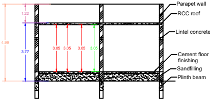
SECTION - AB
