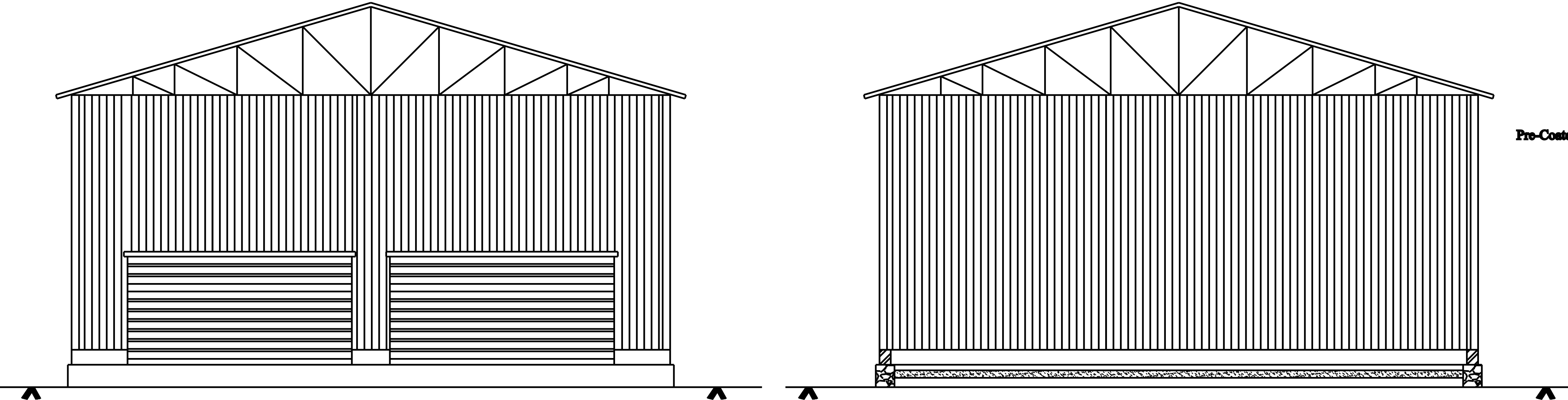
ELEVATION
