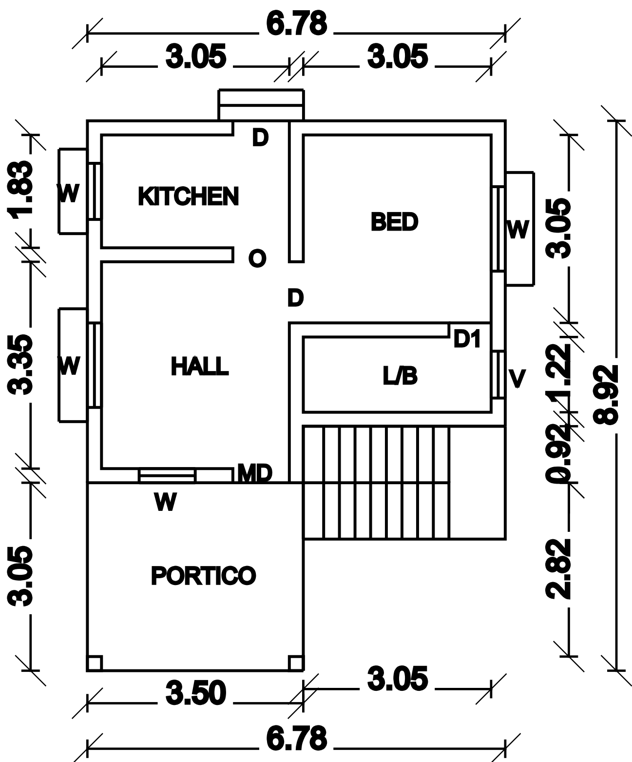
G.F PLAN
