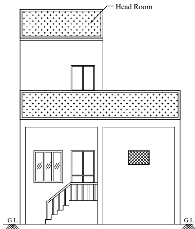
ELEVATION
