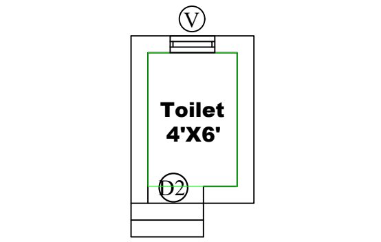
TOILET PLAN
