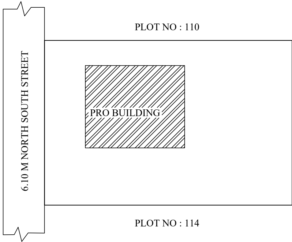
SITE PLAN(SCALE 1:100)
