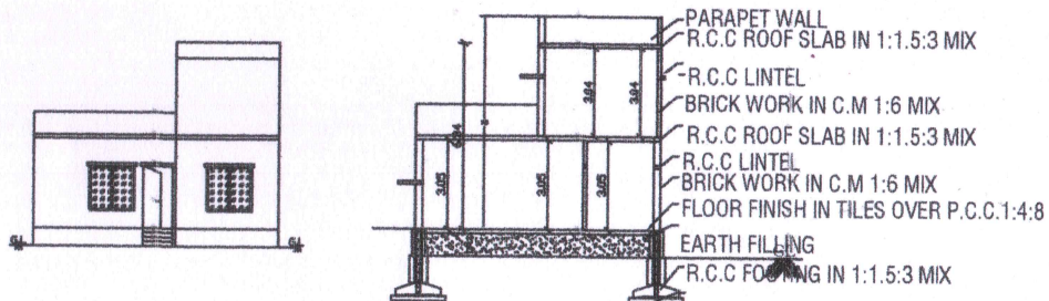
ELEVATION
