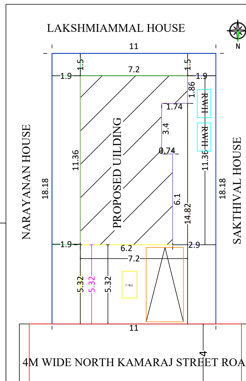
SITE PLAN 1:100 SCALE
