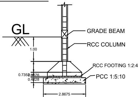
SECTION ON - BB (N.T.S)
