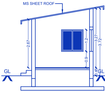
SECTION-A
