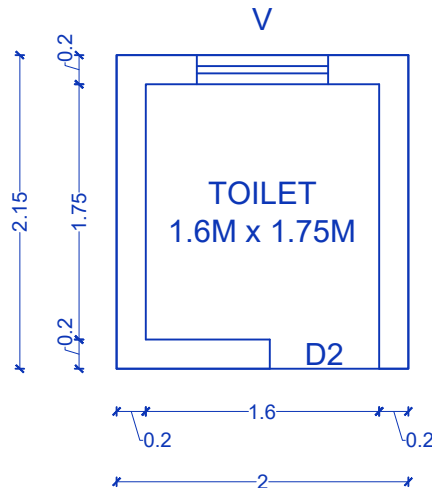
TOILET PLAN
