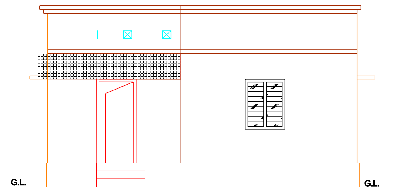
ELEVATION
