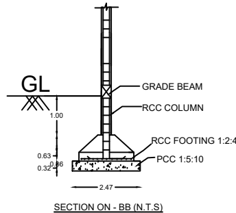
SECTION ON - BB (N.T.S)
