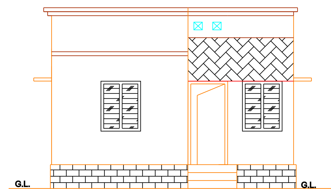
ELEVATION
