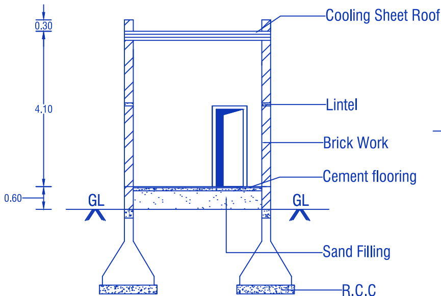
SECTION ON'AB'
