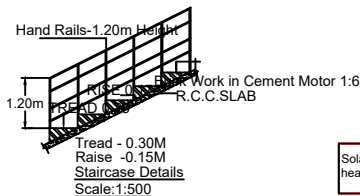
Scale:1:500
