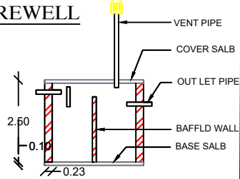
SECTION ON X - Y
