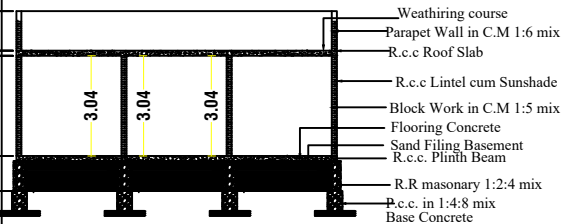
SECTION A-B
