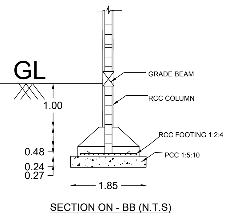
SECTION ON - BB (N.T.S)
