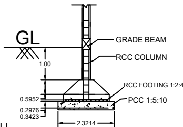
SECTION ON - BB (N.T.S)
