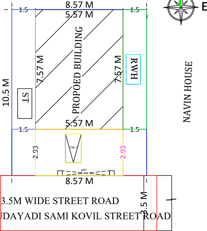
SITE PLAN 1:100 SCALE
