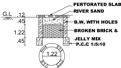
R.W.C.T, PLAN & SECTION
