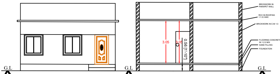
ELEVATION
