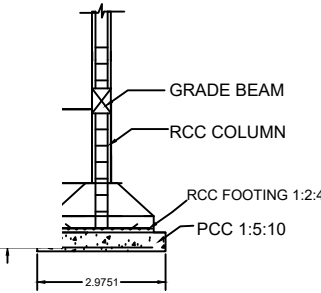
SECTION ON - BB (N.T.S)
