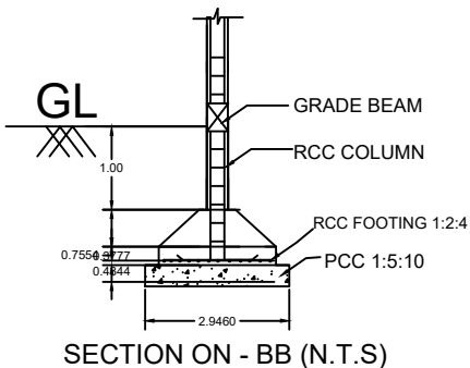
SECTION ON - BB (N.T.S)
