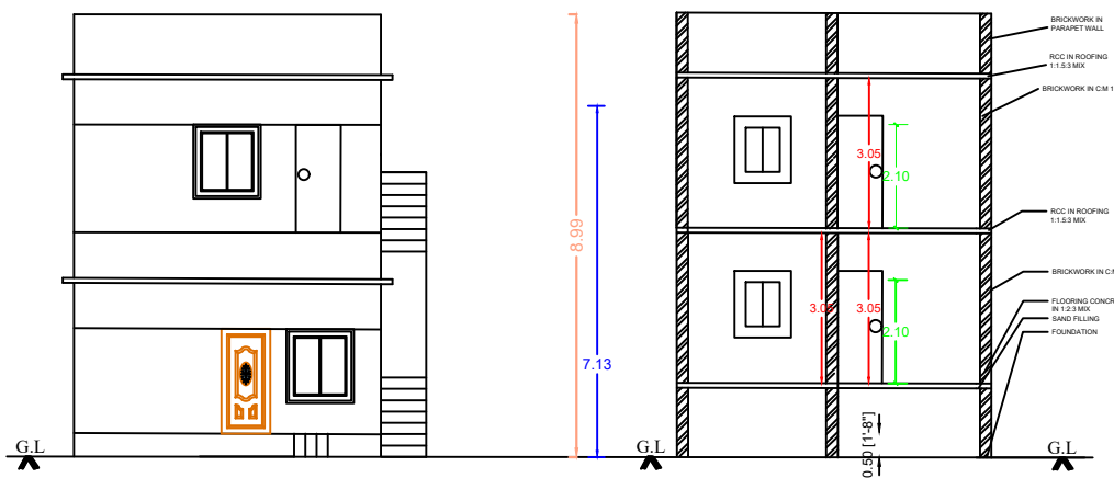
ELEVATION
