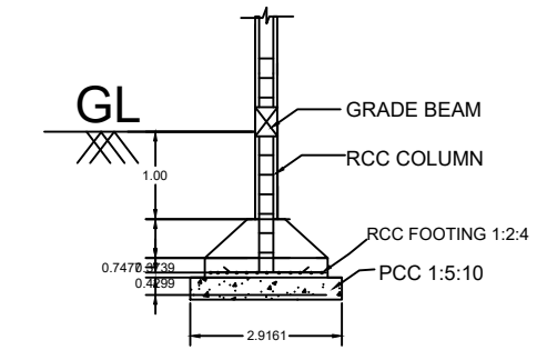
SECTION ON - BB (N.T.S)
