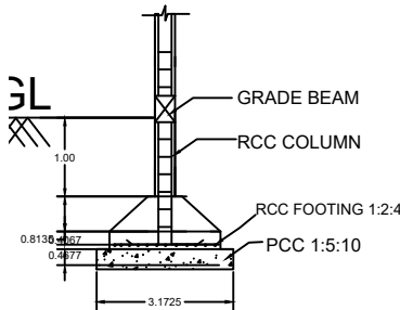
SECTION ON - BB (N.T.S)
