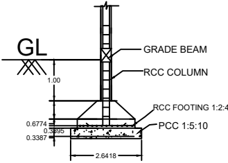
SECTION ON - BB (N.T.S)
