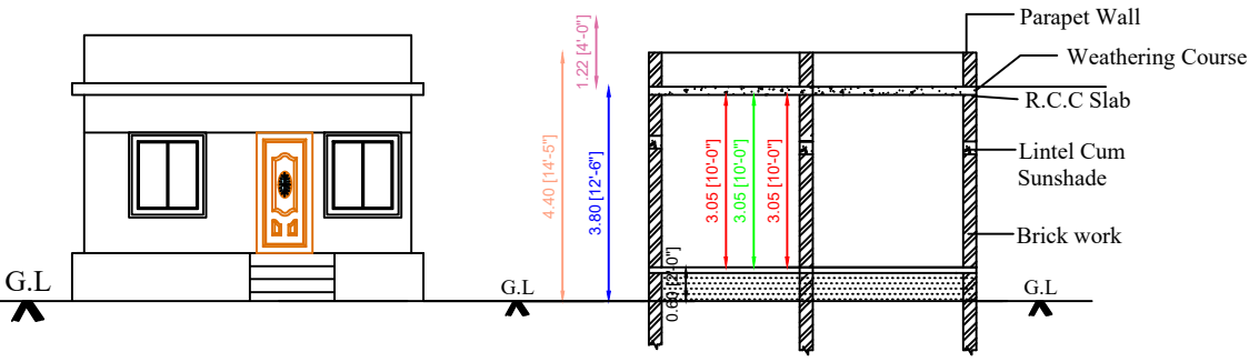
ELEVATION
