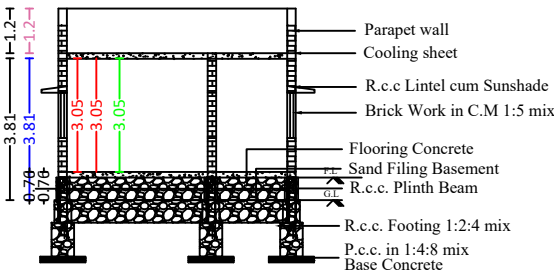
SECTION A-B
