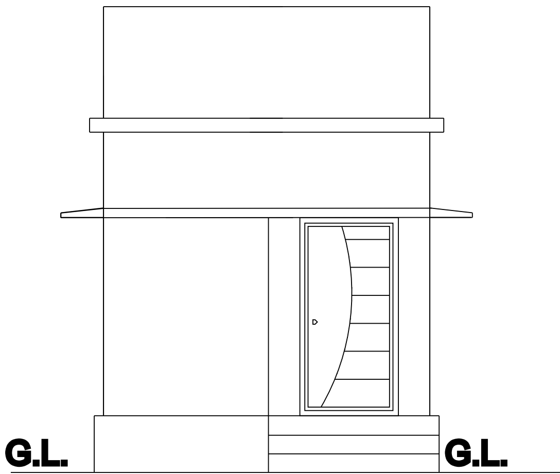
ELEVATION
