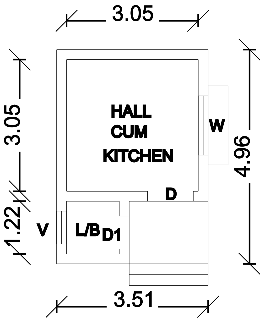
G.F PLAN
