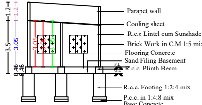
SECTION A-B
