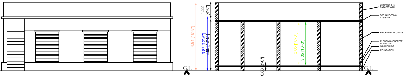
ELEVATION
