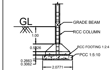
SECTION ON - BB (N.T.S)
