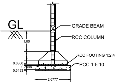
SECTION ON - BB (N.T.S)
